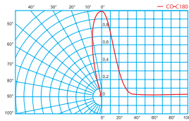
Исполнение «Г 30»
